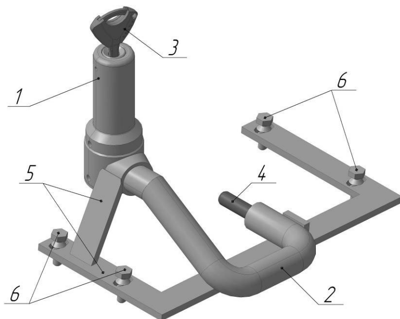
Рисунок 2. Противоугонный механический замок «Гарант Консул» с гибким приводом
