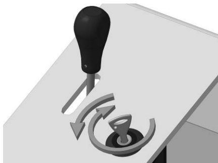
Рисунок 3. Закрывание замка
